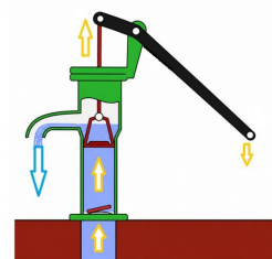
Bovenste klep dicht onderste open
