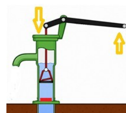
Bovenste klep open, onderste dicht
